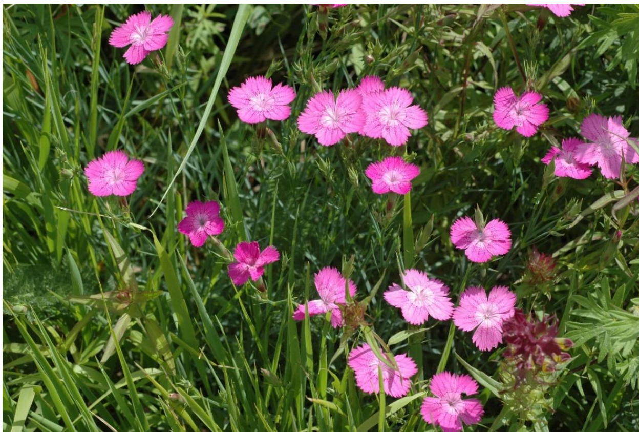
Рис. 3. Dianthus acantholimonooides Schischk. (окр. пос. Макопсе, ущ. р. Неожиданная). Fig. 3. Dianthus acantholimonooides Schischk. (Makopse village, gorge of Neozhidannaya river).
